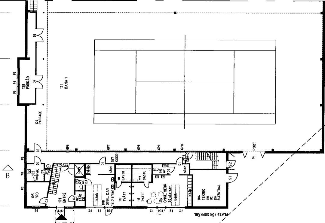
PLAN 1, del av
