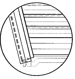
Takfotsdetalj skala 1:20
